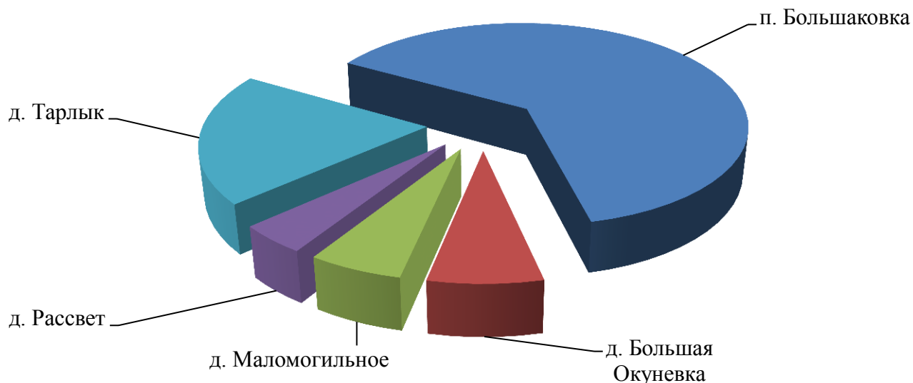
Рисунок 3.1 – Территориальный водный баланс
