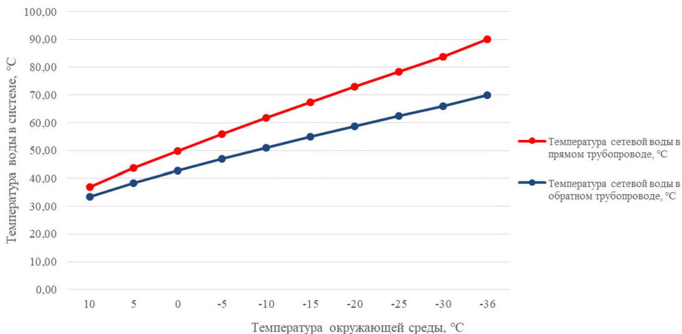
Рисунок 2.2 – График изменения температур теплоносителя (температурный график 90/70°C)
